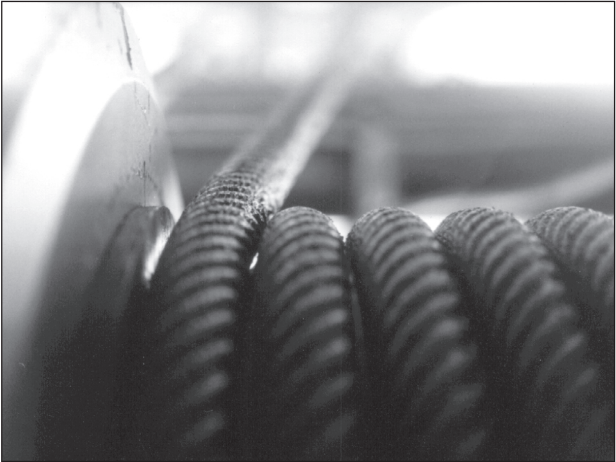
Bild 44: Unter dem Einfluß eines Ablenkwinkels wird das Drahtseil gegen seine Nachbarwindung gezogen. Die Außendrähte werden an der Berührungsstelle beschädigt.
