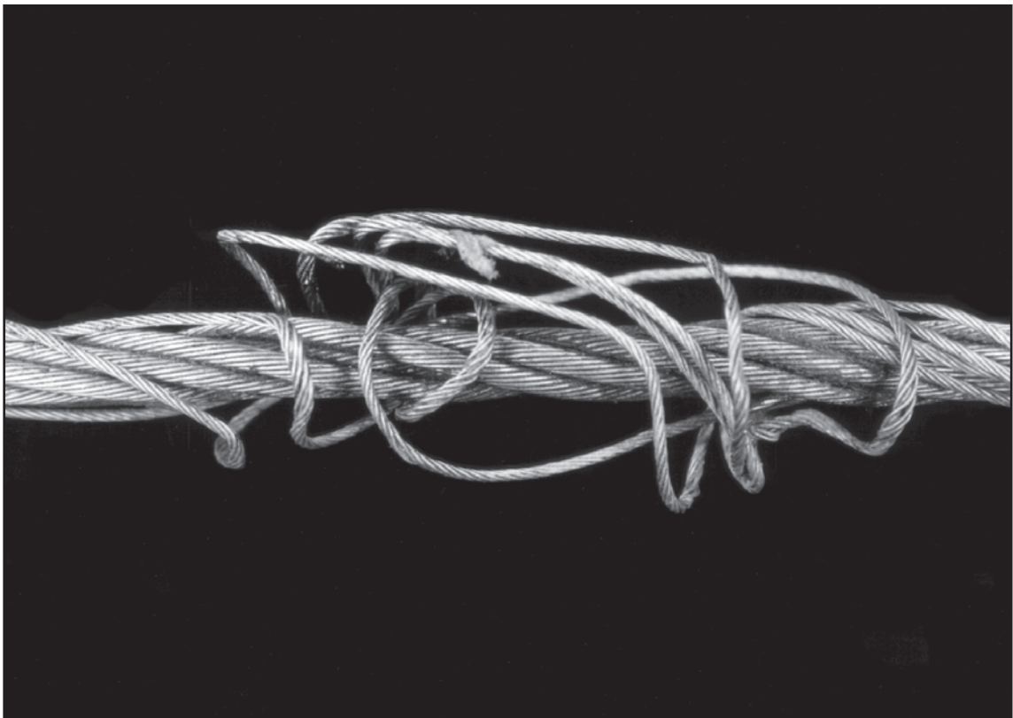
Bild 38: Längenüberschuß der Innenlitzen, verursacht durch Zudrehen des gleichen Drahtseils
