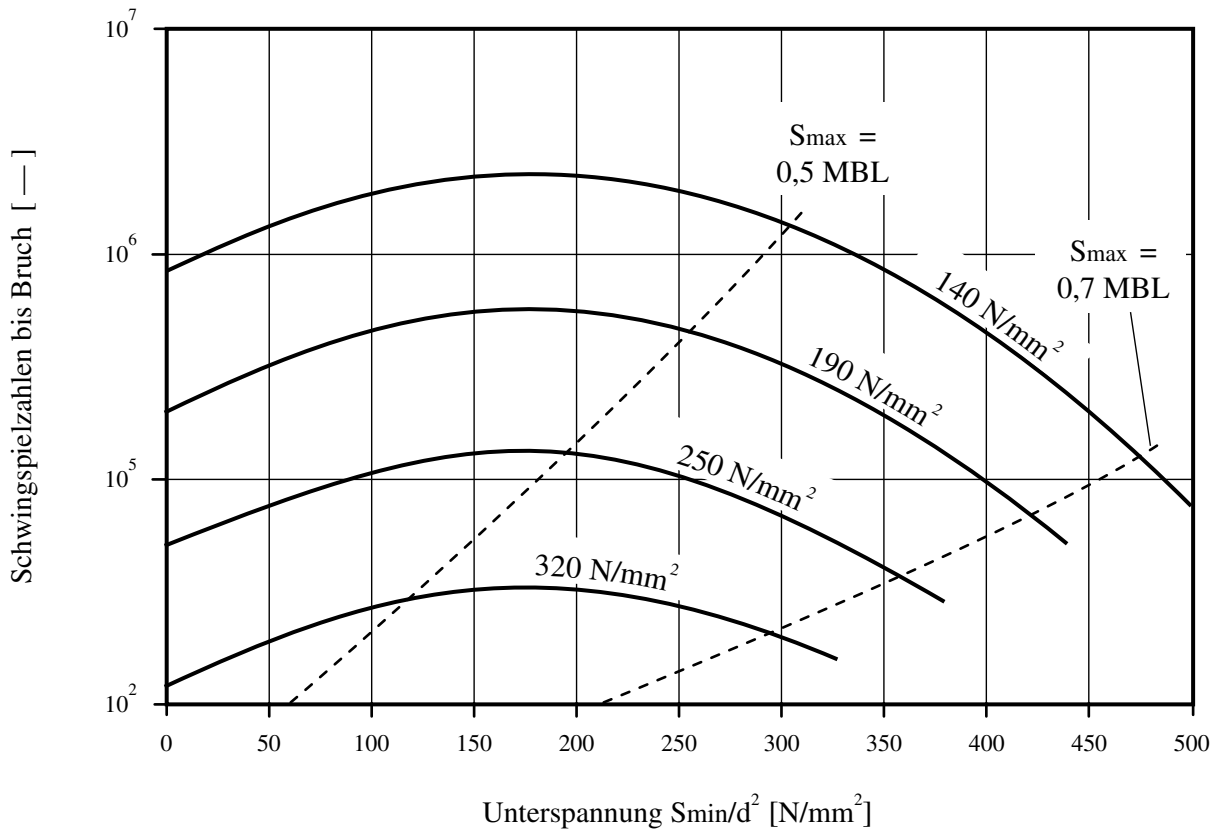
Bild 33: Mit zunehmender Mittelspannung erzielen Drahtseile bis zu einer Gesamtbelastung von 50% ihrer Mindestbruchkraft höhere Schwingenspielzahlen.
