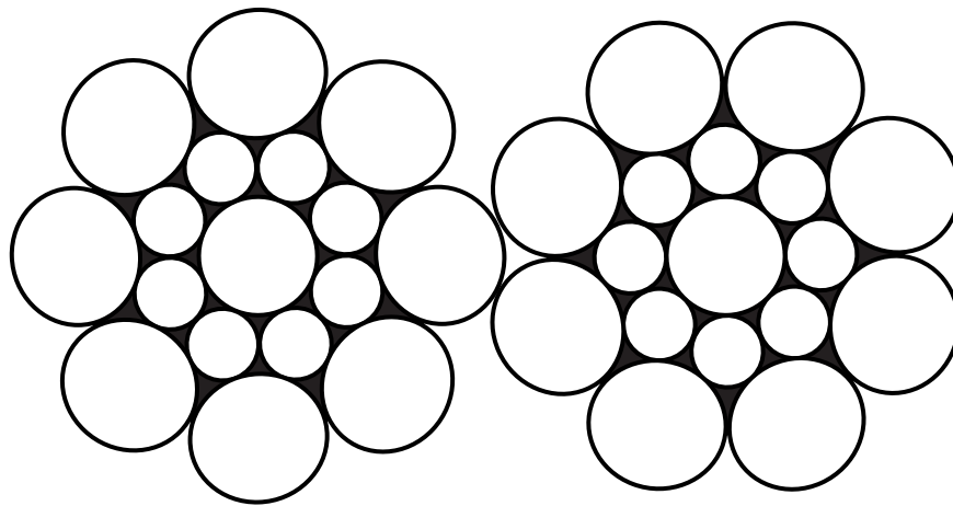
Bild 45: Die Außendrähte zweier benachbarter Windungen eines Kreuzschlagseils können sich ineinander verzahnen.
