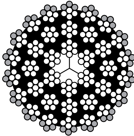
Bild 5: Nur 20% des Metallquerschnittes (grau dargestellt) können visuell begutachtet werden.
