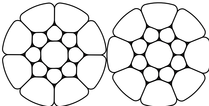
Bild 46: Die Berge und Täler verdichteter Außenlitzen sind abgeflacht und geglättet. Der Metallquerschnitt ist erhöht, um Abrieb und mechanischer Beschädigung besser zu widerstehen.
