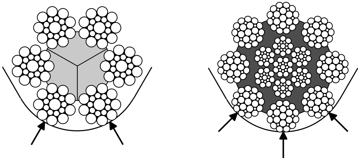
Bild 24: Wegen ihrer größeren Zahl von Auflagepunkten in der Seilrille und den hieraus resultierenden geringeren Pressungen haben 8-litzige Drahtseile (z. B. Casar Strastoplast, rechts) eine höhere Biegewechselfestigkeit als 6-litzige Drahtseile (links).
