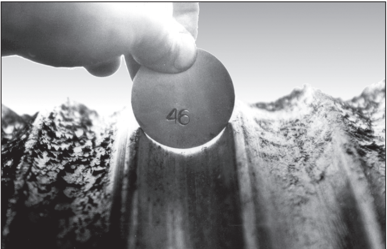
Bild 43: Zu enge Seilrille
